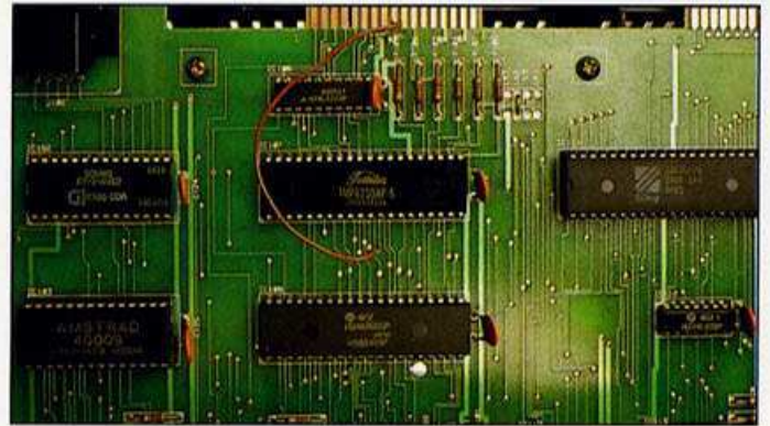
Ein Draht »spendet« dem Centronics-Port das fehlende Bit
